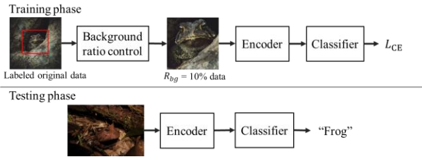
그림 3. 분류 모델 처리 흐름
